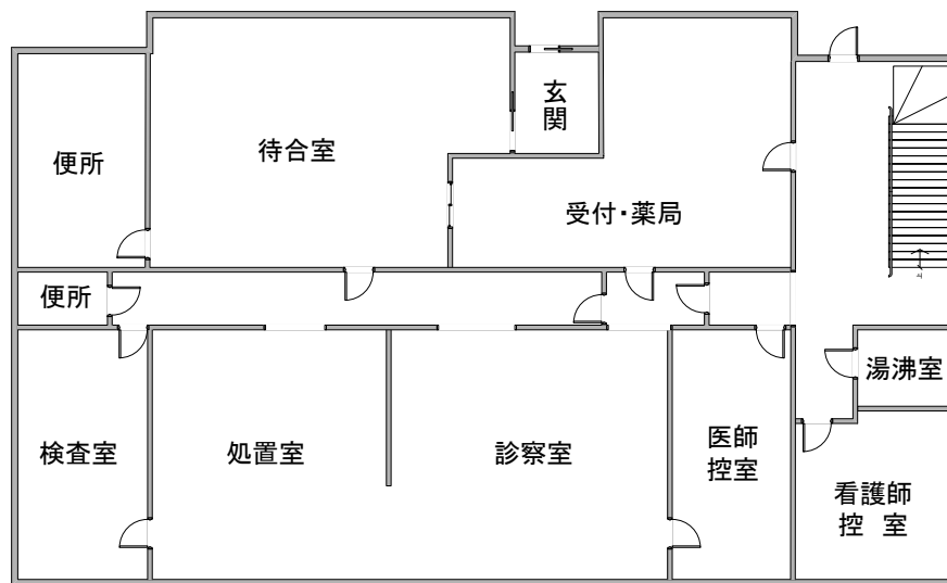
東部休日急病診療所 1 階平面図
