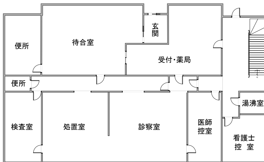
休日急病診療所 1 階平面図
