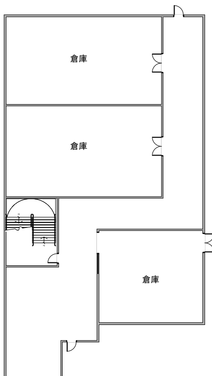
通信指令室棟 1 階平面図
