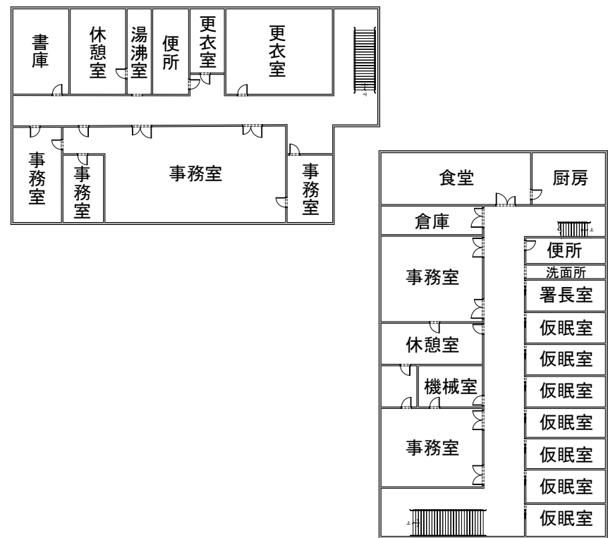
西消防署 2 階平面図
