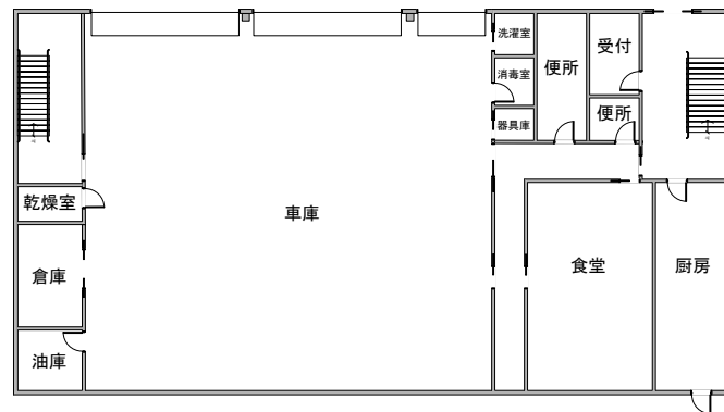
東消防署 2 階平面図
