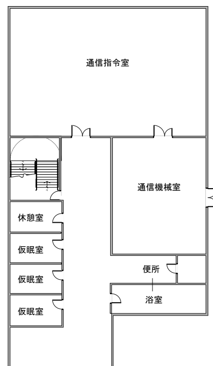
通信指令室棟 2 階平面図
